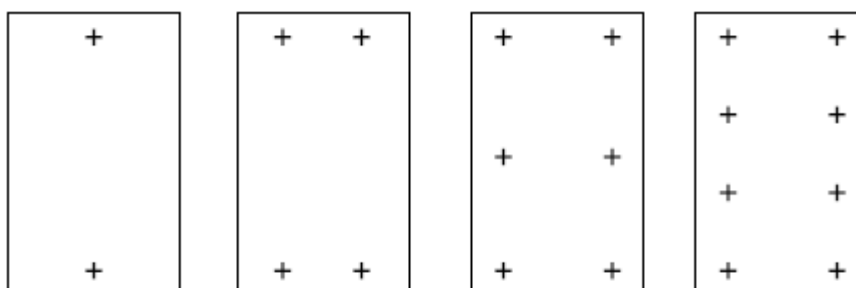
Fig. 2 – Plaatsingspatroon voor de mechanische bevestigingen
